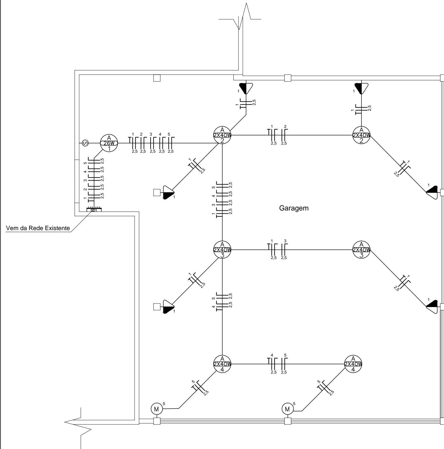
Planta Baixa - Projeto Elétrico
